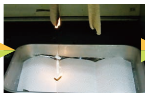
火源を離すと、どちらも繊維自体の火は消えますが、難燃ポリエステルは溶融した繊維が下に垂れできます。
